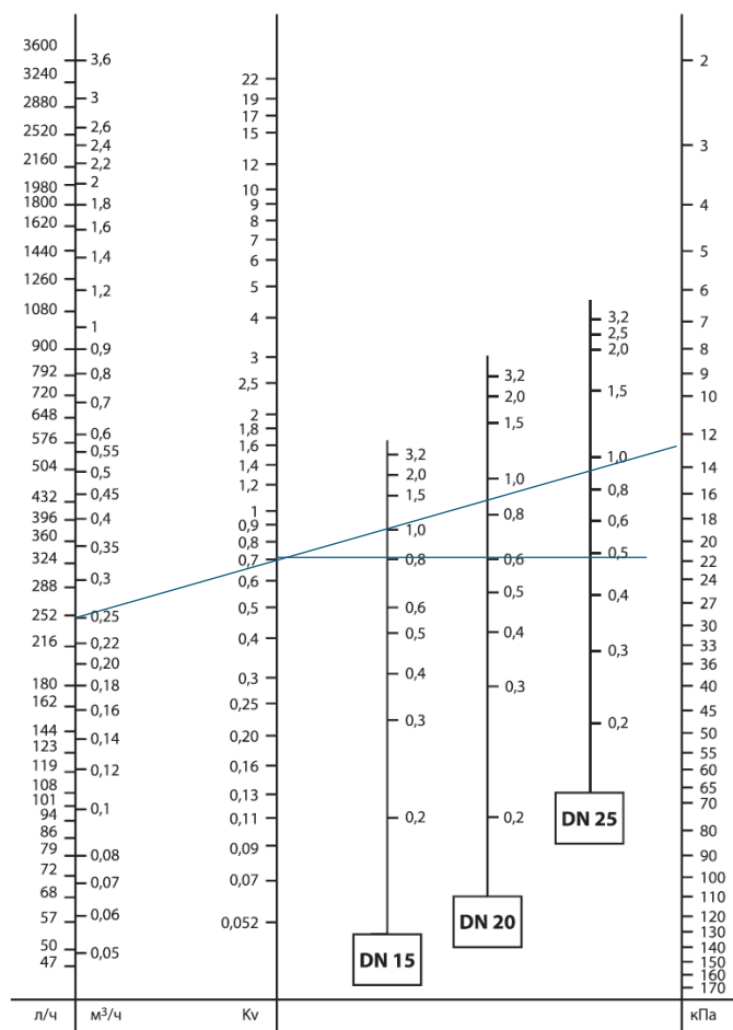
Рисунок 3 – Пример определения предварительной настройки клапана по диаграмме
