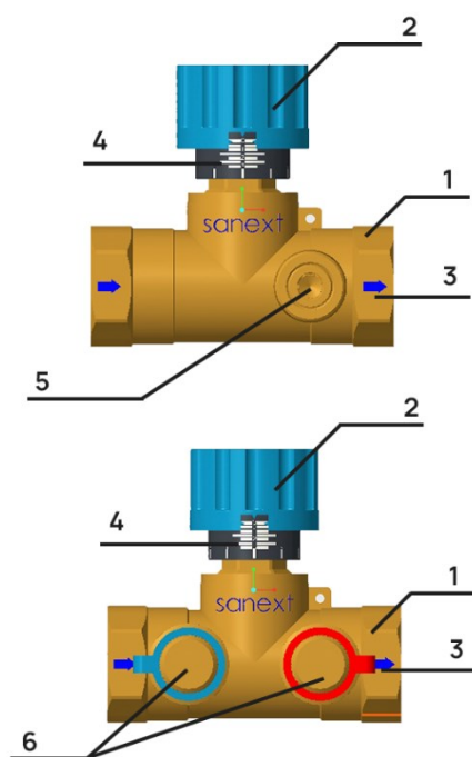
Рисунок 1 – Конструкция клапана STP B
