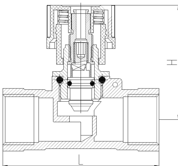
Рисунок 2 – Габаритные размеры
