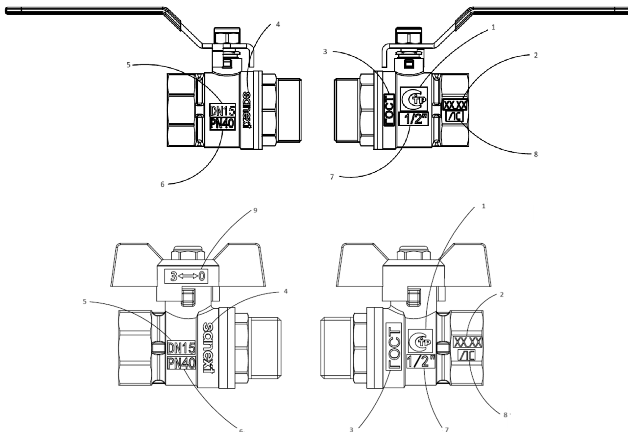
Рисунок 1 – Пример маркировки Шарового крана
