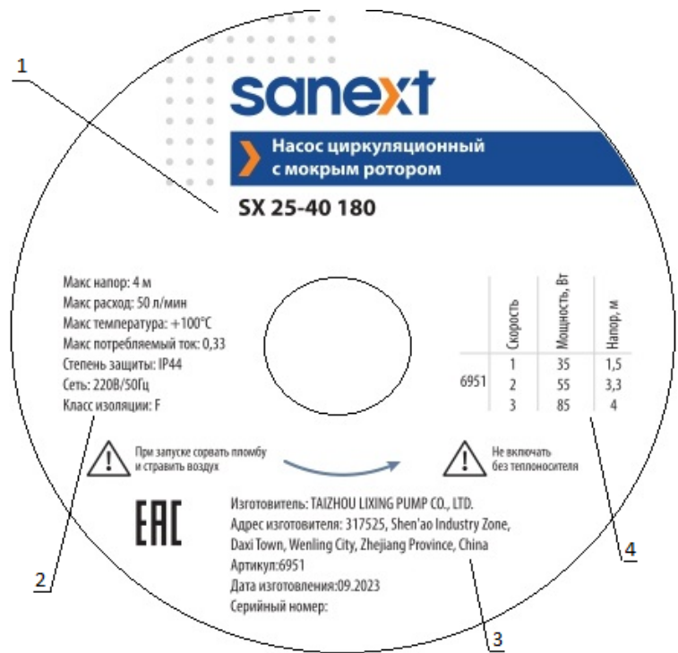
Рисунок 1 – Шильд изделия
