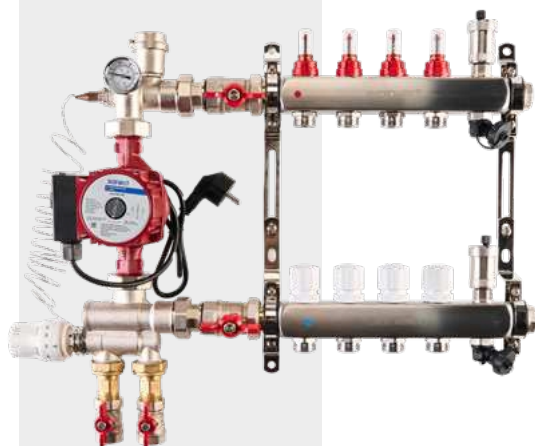
ПКУ SANEXT «Тёплый пол» с насосно-смесительным узлом
