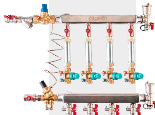
РАСПРЕДЕЛИТЕЛЬНЫЙ КОЛЛЕКТОРНЫЙ УЗЕЛ SANEXT «ЭТАЖНЫЙ-DSI SF»
