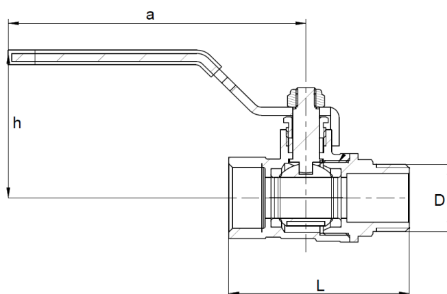
Рисунок 3. Габаритные размеры арт. 8764, 8765, 8766
