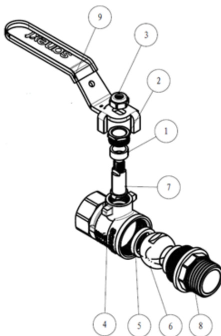
Рисунок 2 – Шаровый кран ВН ДУ32-50 (арт 8764, 8765, 8766)
