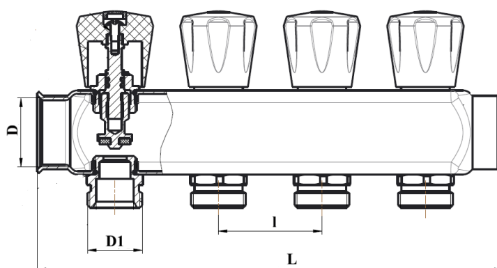
Рисунок 1 – Габаритные размеры
