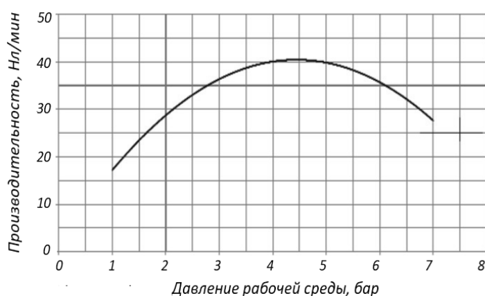
Рисунок 2 – График производительности
